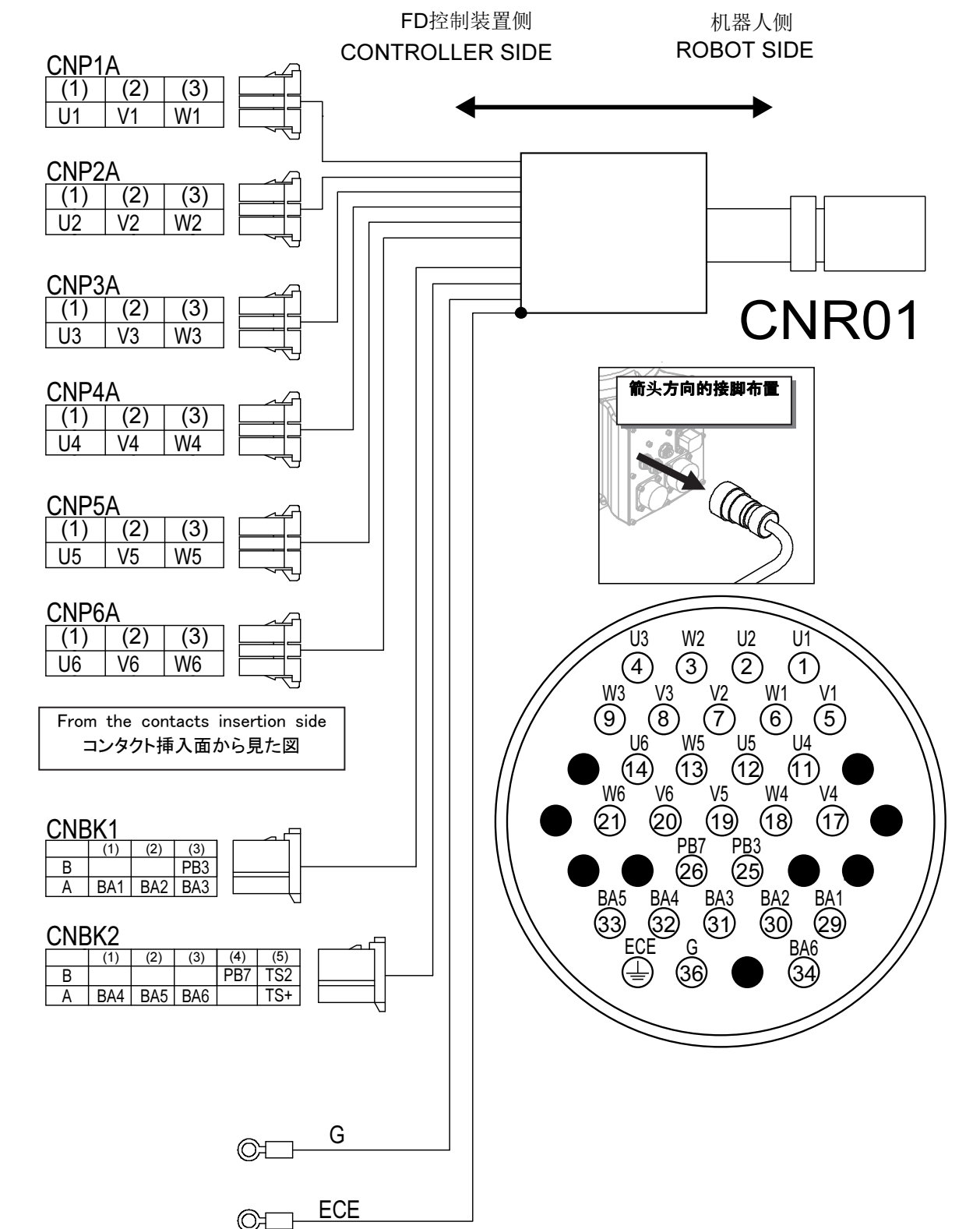
FD控制装置用 缆线组连接(1) CNR01
