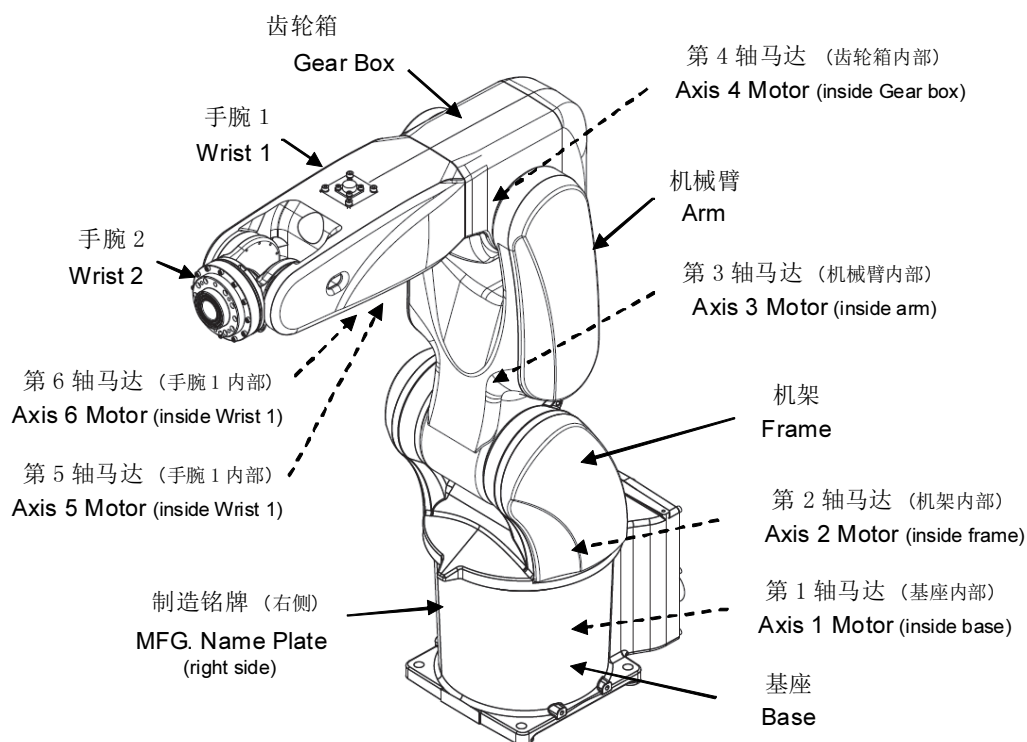
动作轴名称和动作方向
