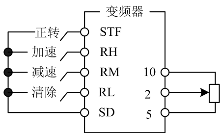
远端控制设定的接线图示例
