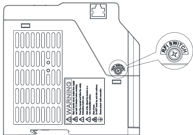
框架 A/B
