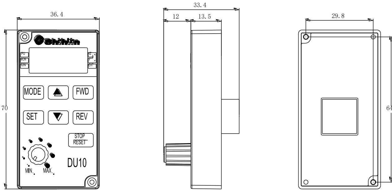
<外形尺寸图>
