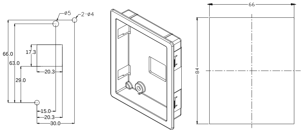
<盘面安装开孔尺寸图><法兰式安装开孔尺寸图(注)>
