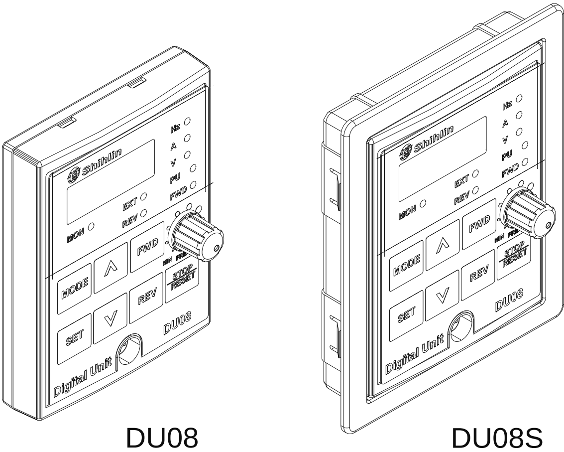
DU08 外观图
