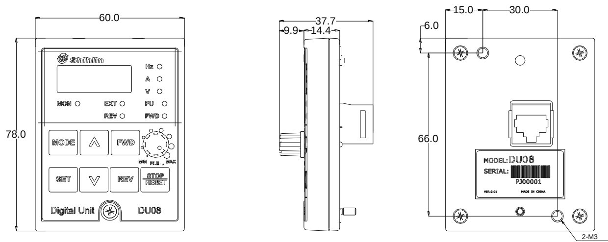
<外形尺寸图>
