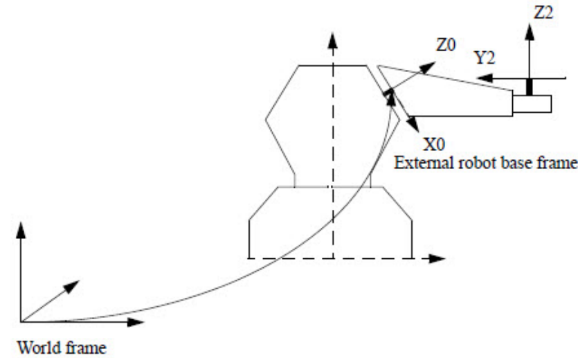
图52：运用通用运动模型的ORBIT_160B机械臂的基准坐标系
