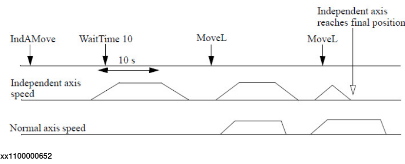
图33：逐步操纵独立轴
