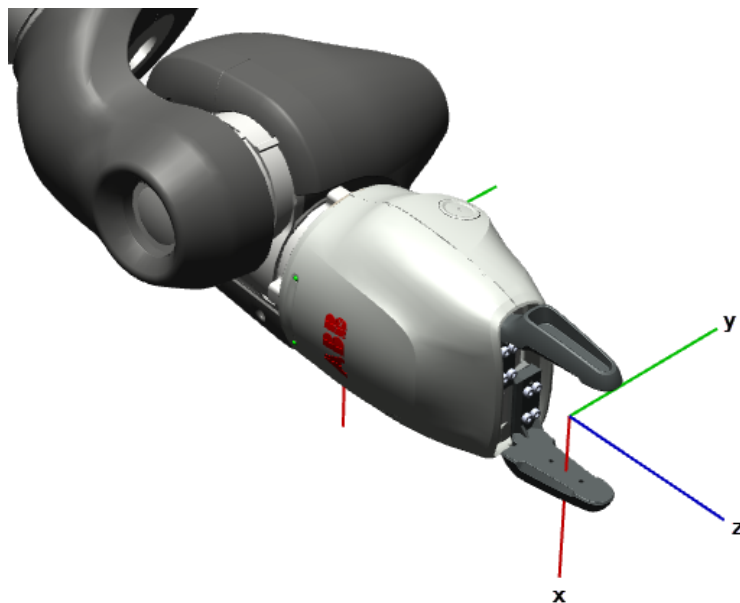
图19：工具坐标系是相对于腕坐标系而定义的，此处所示为夹具坐标系。
