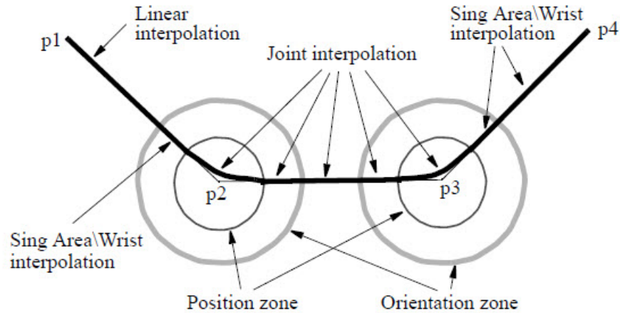
图30：从一种插补法转变为另一种时的插补情况。 p1 和 p2 之间，设定用直线插补； p2 和 p3 之间用关节插补； p3 和 p4 之间用Sing Area\Wrist插补。
