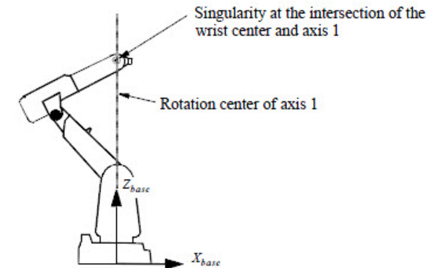
图54：腕中心和轴1汇集时出现臂奇异点
