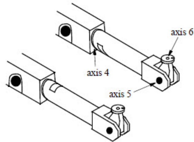
图43：到达相同位置和方位所用的两种不同腕配置。在上臂的前端指向上方的配置（下图）中，轴4、轴5和轴6旋转180度，就可获得上臂的前端指向下方的配置（上图）。
