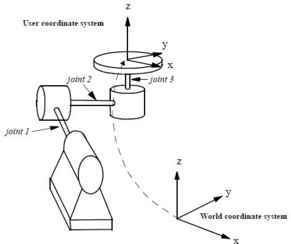
图15：按3轴外部机械单元移动而定义的用户坐标系。
