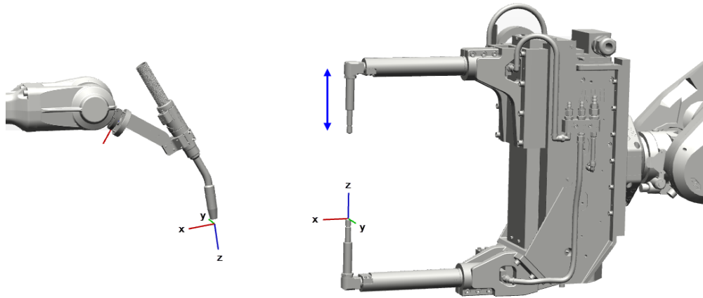
图18：按通常情况定义的弧焊焊枪（左）和点焊焊枪（右）坐标系
