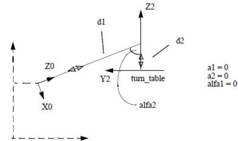
图51：运用通用运动模型的ORBIT 160B机械臂的运动结构
