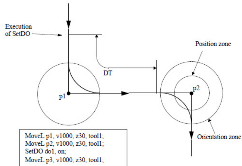
图37：到达最大区域前执行飞越点后的某一逻辑指令。
