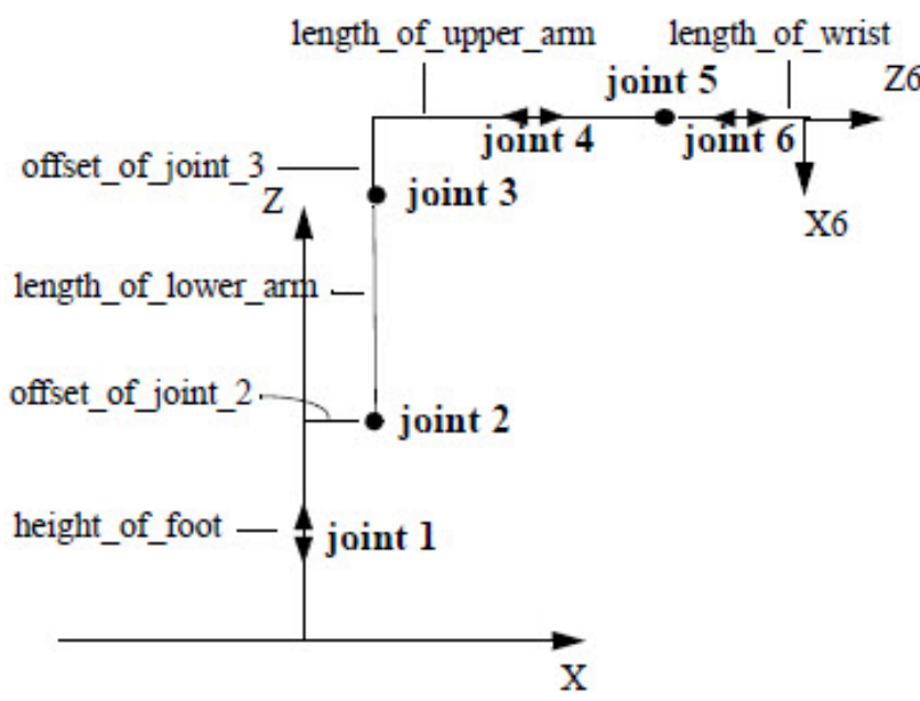
图46：IRB 1400机械臂的运动结构
