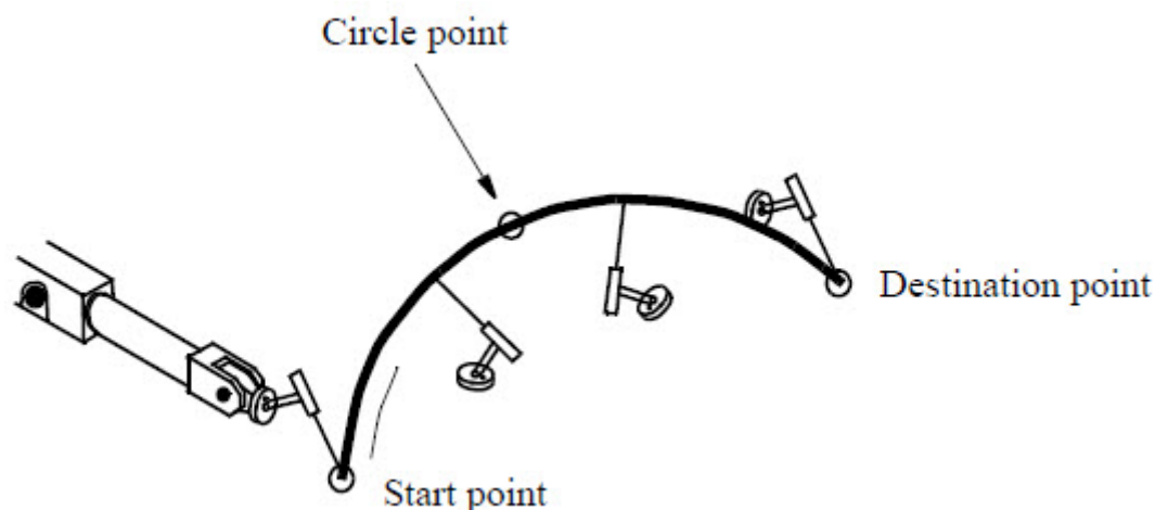
图25：通过定义起点相反方向的圆周点的姿态，利用长姿态曲线实现的圆弧插补。
