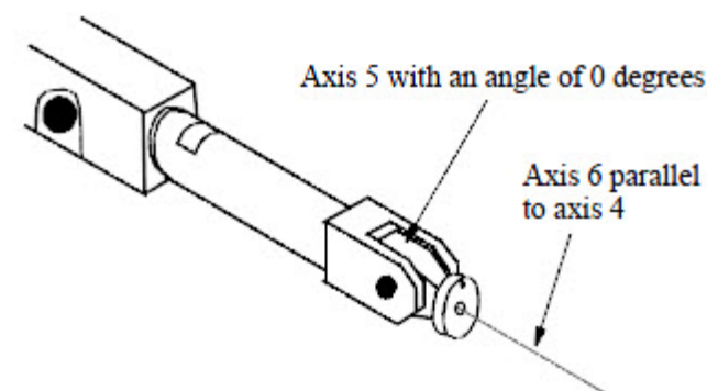
图55：轴5角度为0时出现腕奇异点
