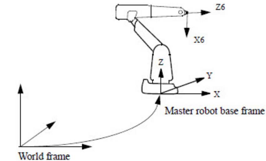
图47：主机械臂的基准坐标系
