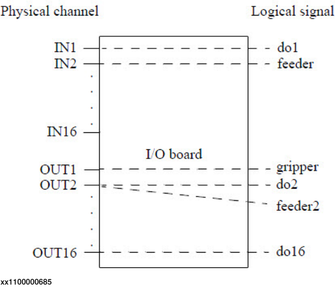
图57：为能使用I/O单板，必须为其通道提供逻辑信号。在上述示例中，实体输出2连接至两个不同的逻辑信号。而另一方面，IN16却没有逻辑信号，因此不能用。
