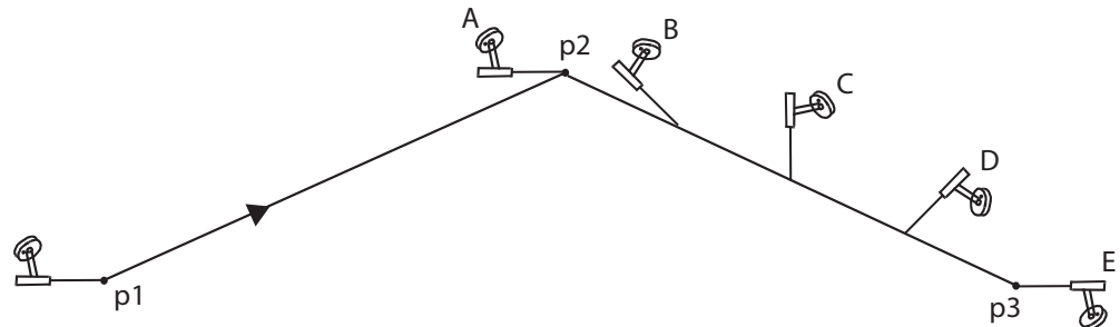
图29a：如将工具方位不同的三个位置设定为停止点，则将照此执行程序。
