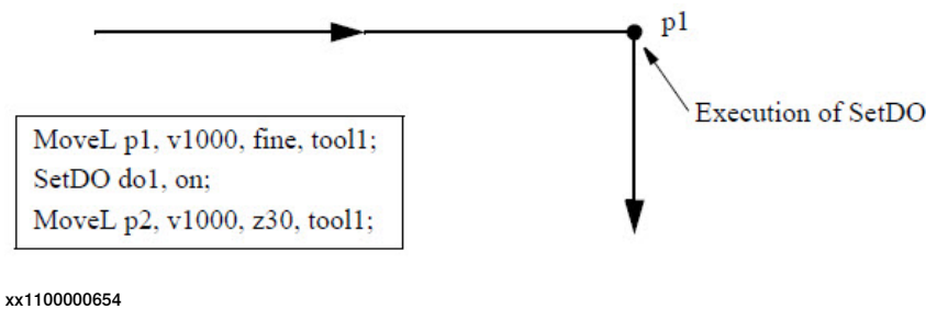
图35：在未到达终点位置前，都不能执行停止点后的逻辑指令。
