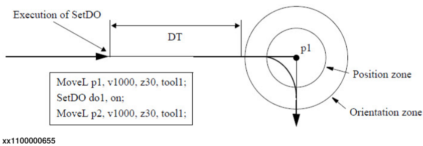
图36：到达最大区域前执行飞越点后的某一逻辑指令。
