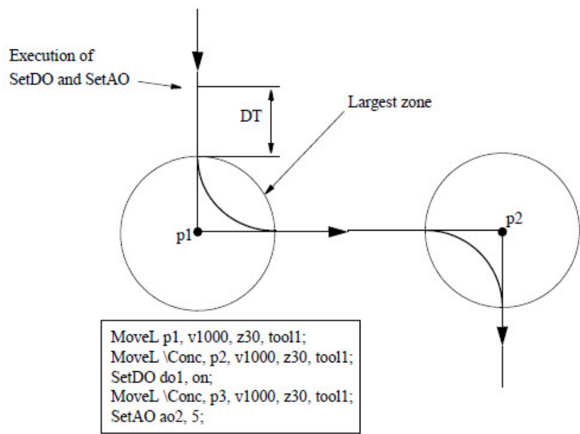
图40：若连续为带参数\Conc的多个定位指令编程，则在执行第一个位置的同时就开始执行所有相连的逻辑指令。
